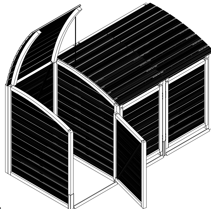
Isometrie Vorderansicht - eine Box geöffnet
